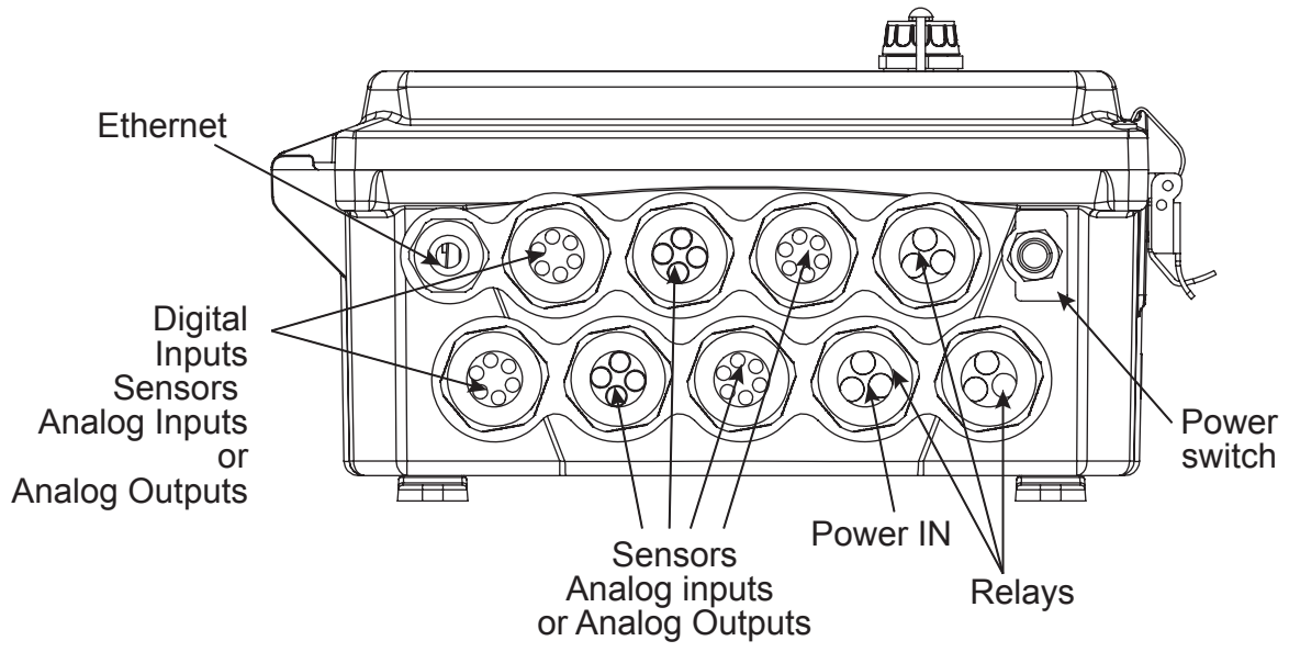
Figure 1 Conduit Wiring
